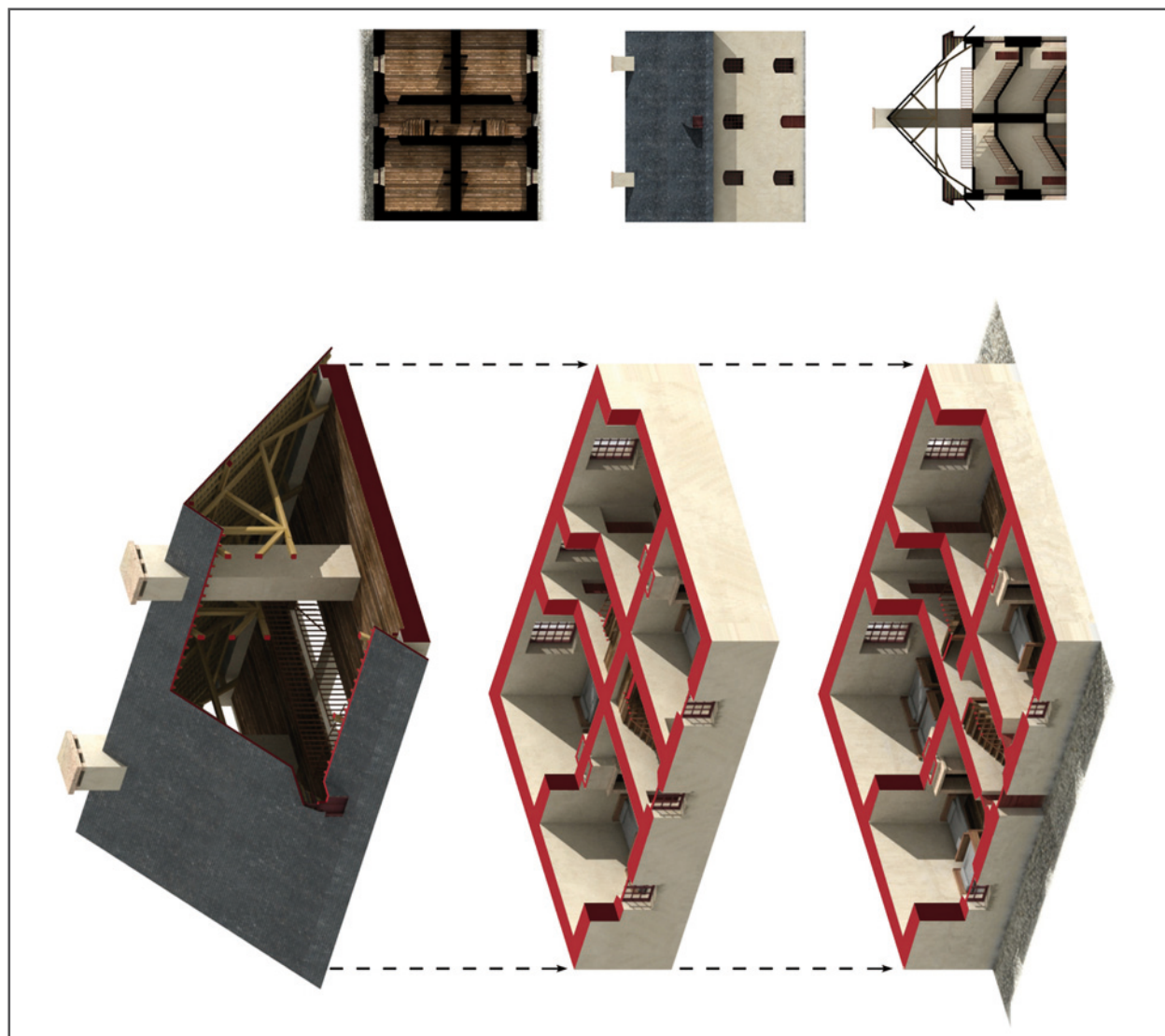
▲ Document 13 : Axonométrie en écorché d'une caserne modulaire selon le modèle de Vauban
